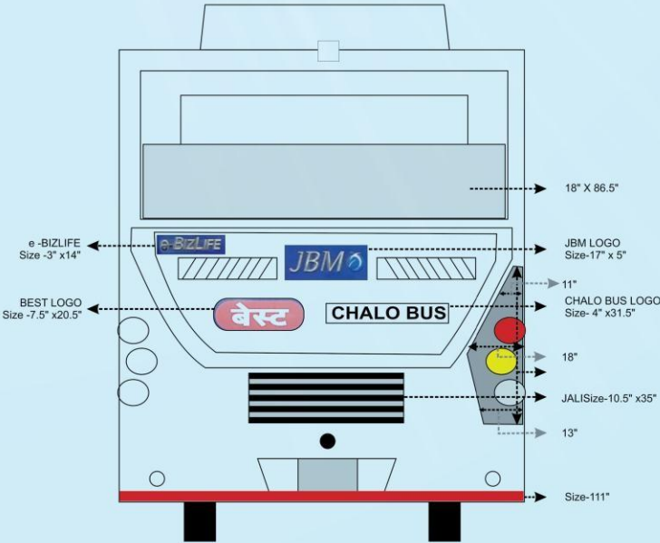
JBM BUS - BACK SIDE
